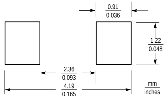
SOT-23
