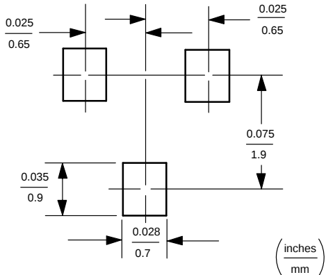
SC-70/SOT-323
