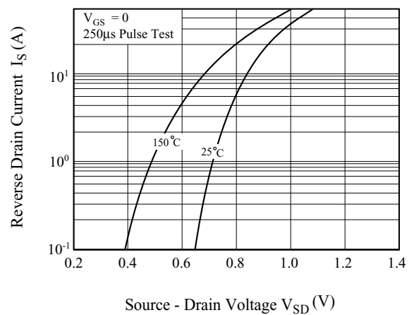
Fig 6. I_{DR} - V_{DSF}
