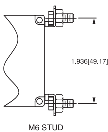
M6 STUD
