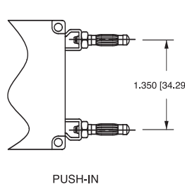
PUSH-IN STUD
