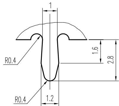
K DETAIL 2 : 1
