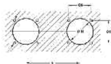
Panel cutout / Perçage panneau
