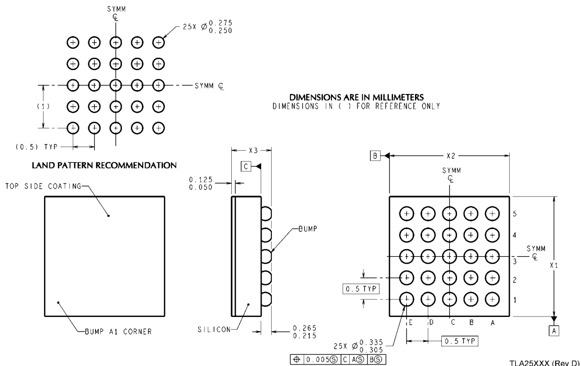
TLA2511A: Micro SMD-25 Package
