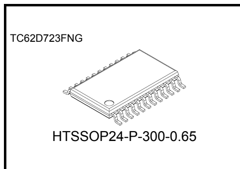
Weight HTSSOP24-P-300-0.65 : 0.10 g (Typ.)
