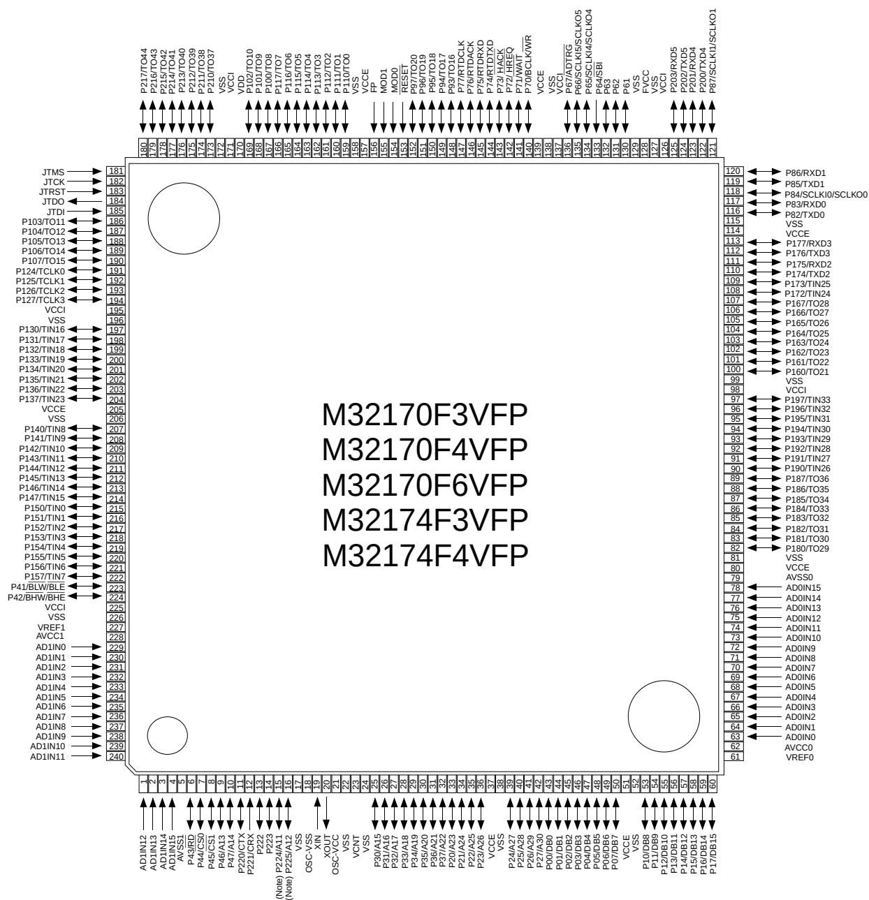
Package 240P6Y-A
