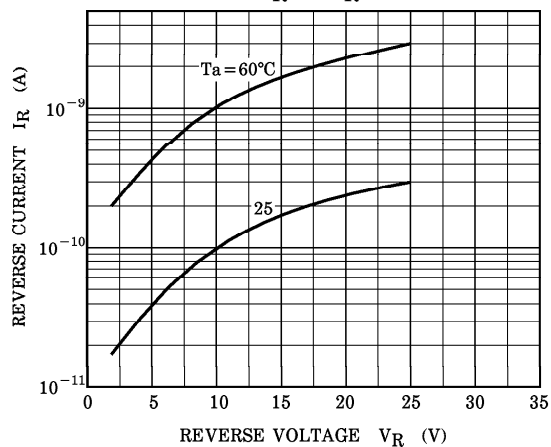
I_R - V_R
