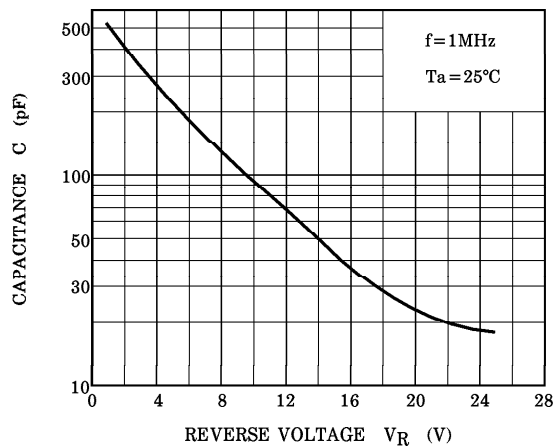
C - V_R
