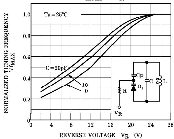
f/f_{\text{MAX}} - V_R
