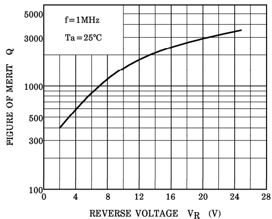
Q - V_R
