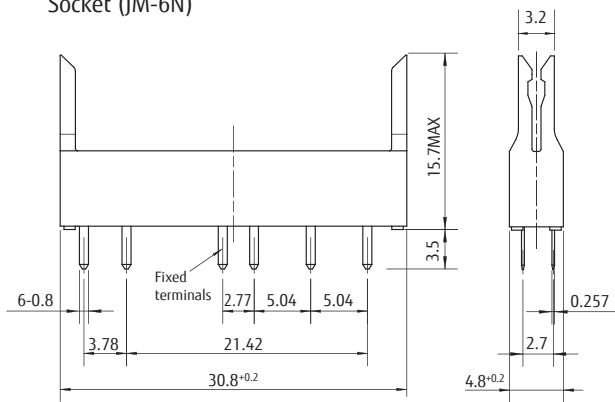
Socket (JM-6N)
