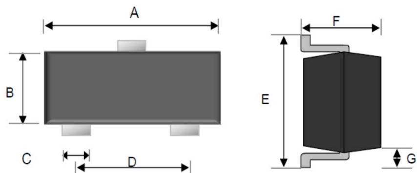
SOT-23
