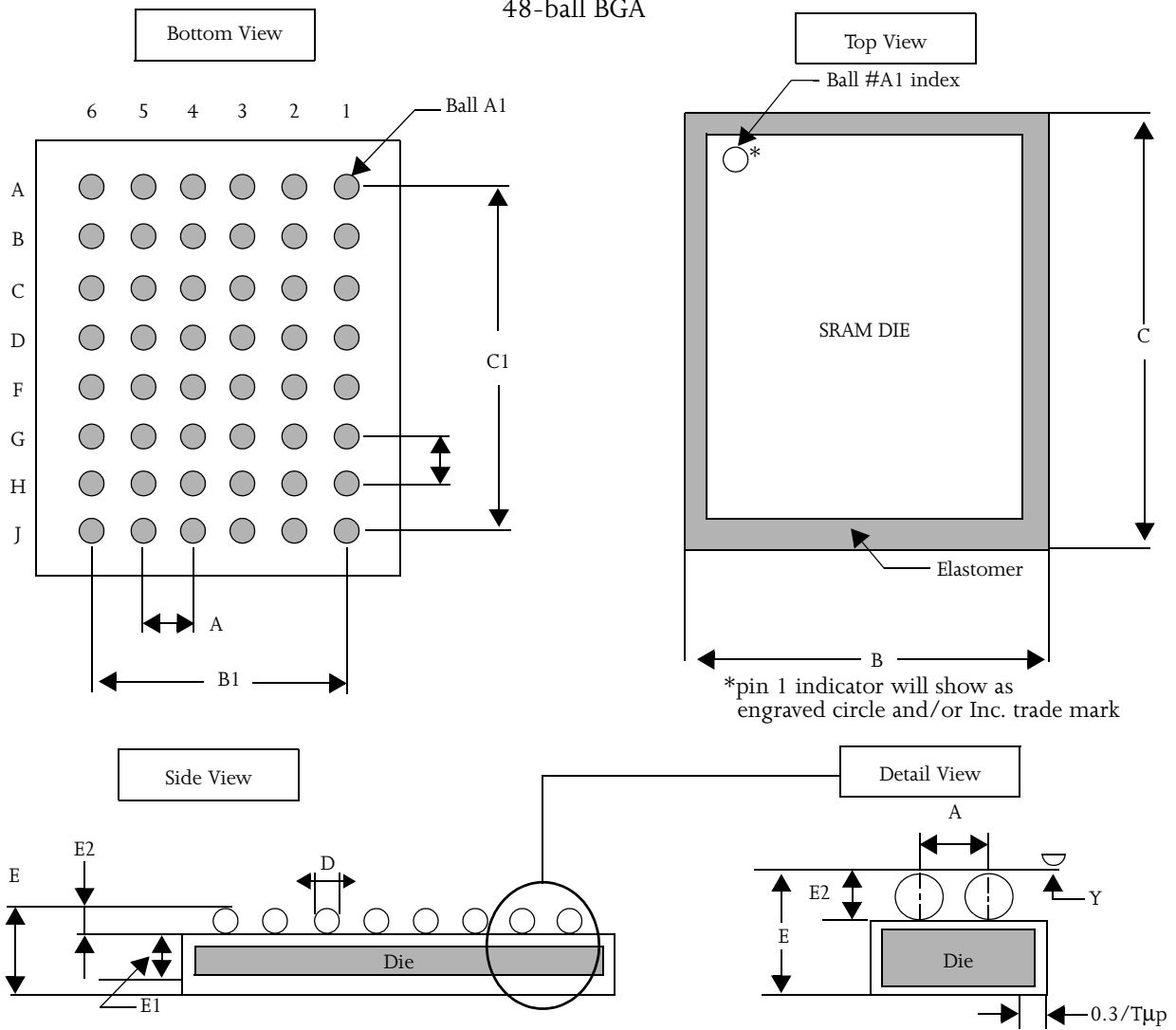
48-ball BGA
