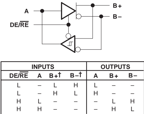
TRANSCIEVER
