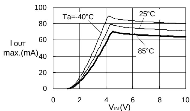
S-817A11A
