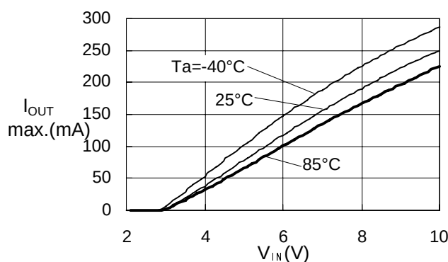
S-817B30A
