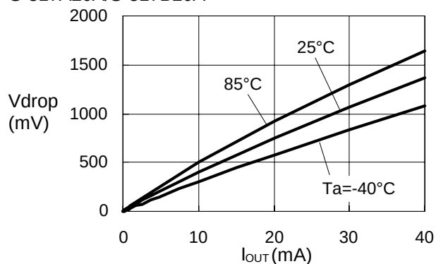
S-817A20A/S-817B20A
