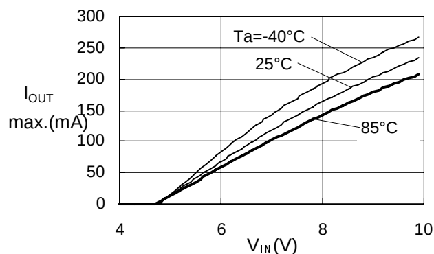
S-817B50A
