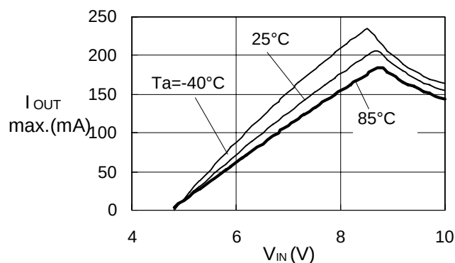
S-817A50A
