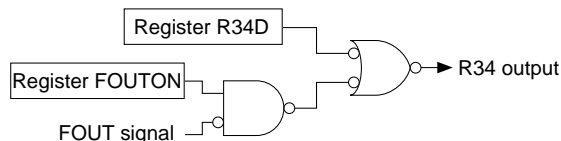
Fig. 5.6.5.11 Configuration of R34
