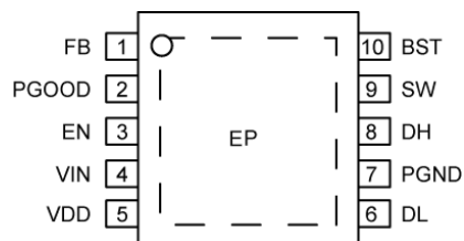
10-Pin ePad MSOP (MME)
