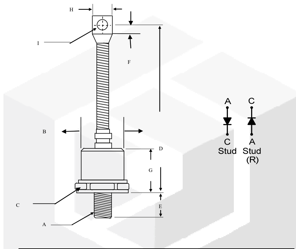
DO-9 (DO--205AB)
