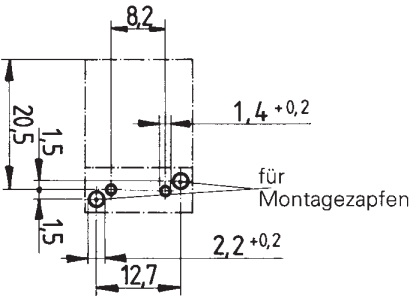
Bohrplan für Buchsenteil
