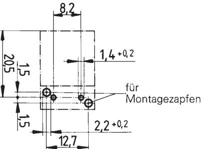
Bohrplan für Steckerteil
