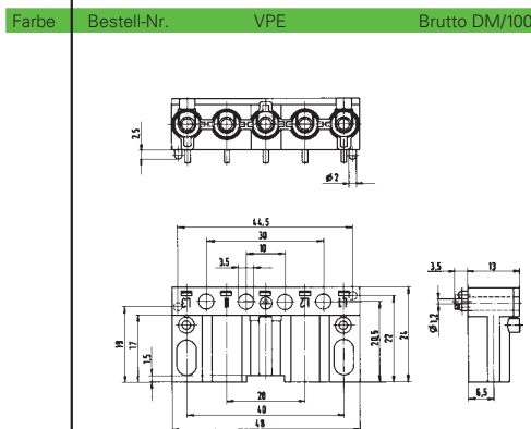
Lochschablone für abgewinkelte Steckverbinder
