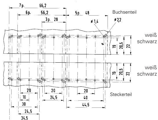
Lochschablone für abgewinkelte Steckverbinder
