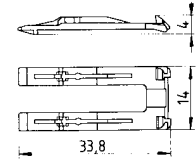
Verriegelungsschieber für Buchsen- und Steckerteile
