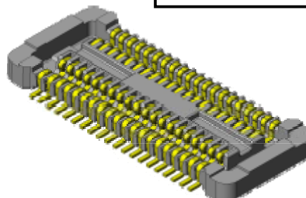
Receptacle
