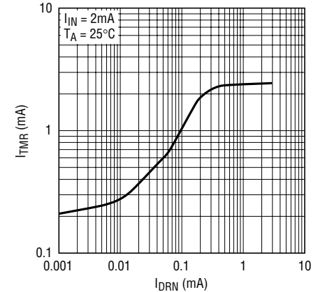
I_{TMR} vs I_{DRN}
