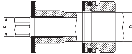
Darstellung für Litzenbündeldurchmesser d und Leitungsaußendurchmesser D
