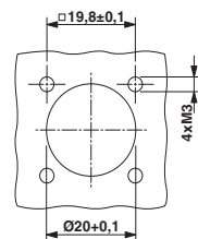
Einbaumaße: SF-.EP1N8AA200
