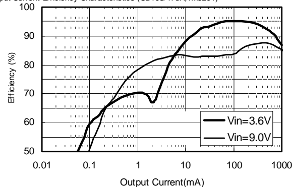
(4) S-8521D30MC
