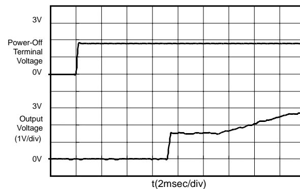
S-8521C30MC (Vin:9.0V)
