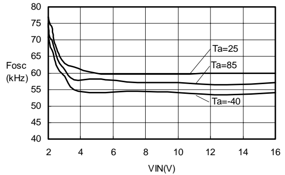
Fosc-VIN S-8520/21(Fosc:60kHz)
