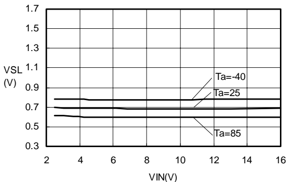
VSL-VIN S-8520/21
