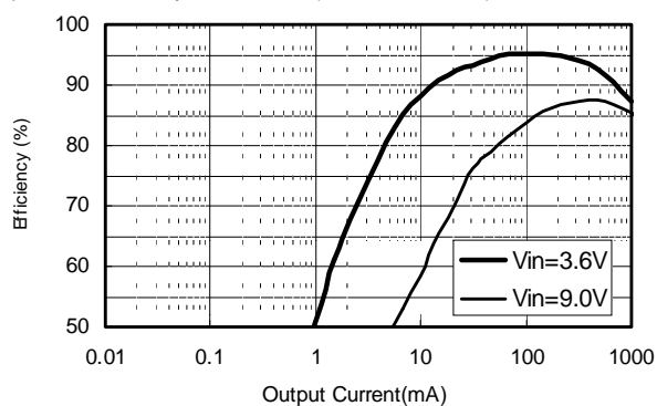
(3) S-8521B30MC
