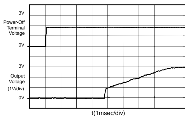
S-8520C30MC (Vin:3.6V)
