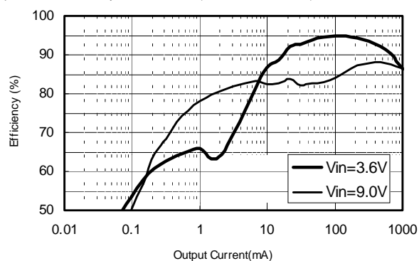
(5) S-8521D30MC
