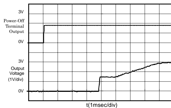
S-8520C30MC (Vin:9.0V)
