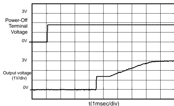
S-8521A30MC (Vin:3.6V)
