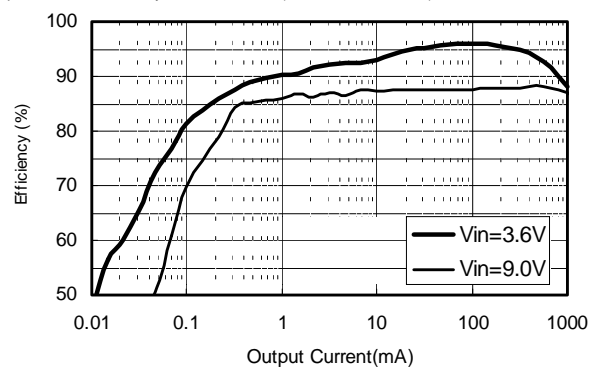
(7) S-8521B50MC
