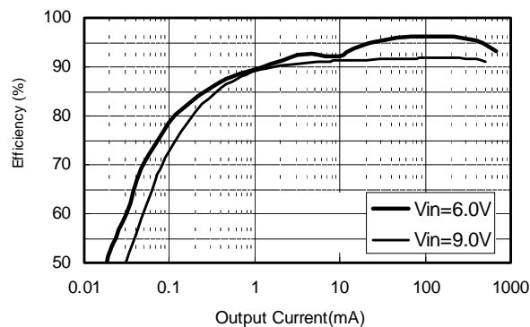
(8) S-8521D50MC
