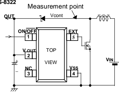
S-8322
