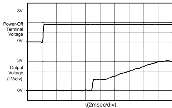
S-8521C30MC (Vin:3.6V)
