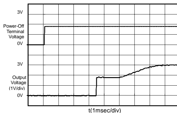
S-8521A30MC (Vin:9.0V)
