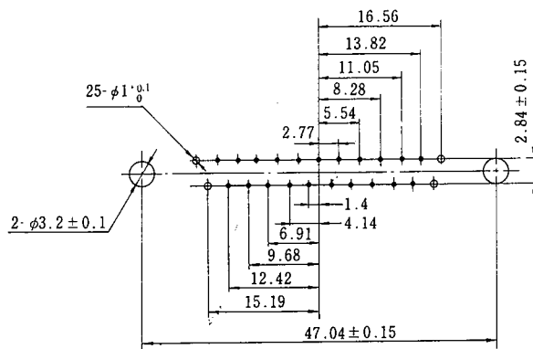
SDBB-25
