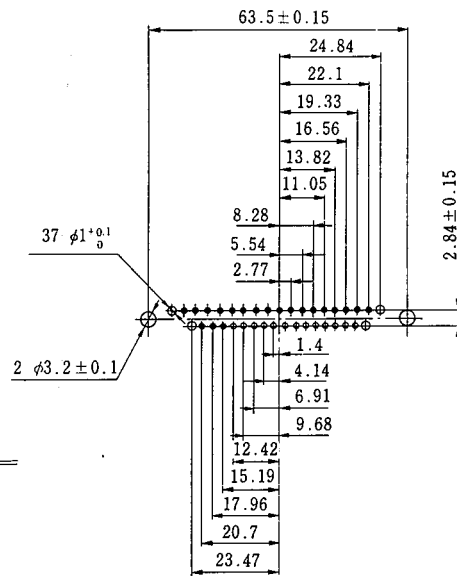
SDCB-37
