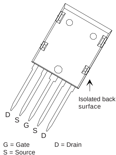
ISOPLUS i5-Pak™ (IXTL)
