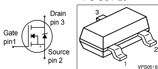
PG-SOT-23
