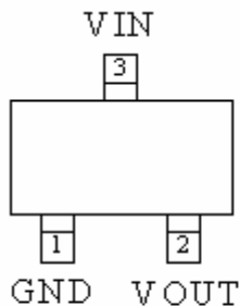
SOT-23-3LA
