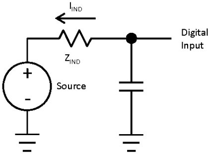
Figure 2. 5 V Tolerant Input IIND Parameter
