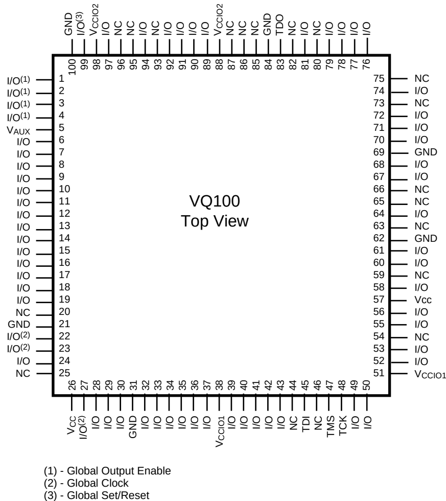
Figure 12: VQ100 Package
