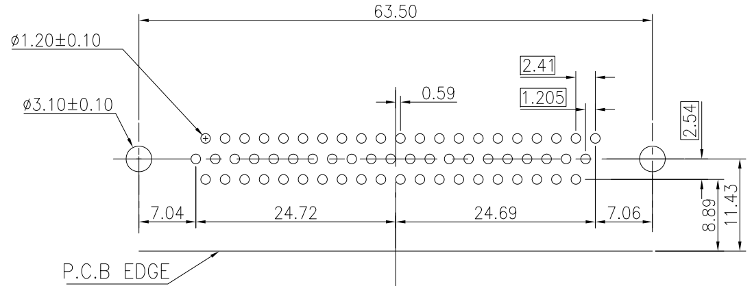
P.C.B LAYOUT(FOR 62P)
