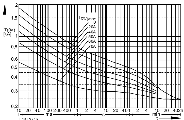
Bild / Fig. 16 Überstrom / Overload on-state current I_{T(OV)} = f(t) Luftselbstkühlung / Natural air-cooling, t_A = 45^\circ\text{C} Kühlkörper / Heatsink: K0.55-M12-A Parameter: Vorlaststrom / Pre-load current I_{TAV(vor)}
