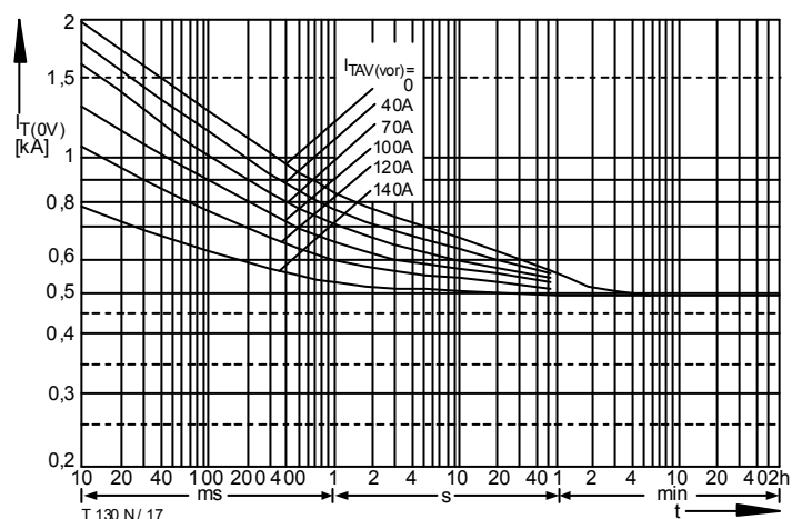
Bild / Fig. 17 Überstrom / Overload on-state current I_{T(OV)} = f(t) Verstärkte Luftkühlung / Forced air-cooling, t_A = 35^\circ\text{C} Kühlkörper / Heatsink: K0.55-M12-A, V_L = 50 l/s Parameter: Vorlaststrom / Pre-load current I_{TAV(vor)}
