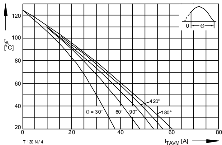
Bild / Fig. 4 Höchstzulässige Kühlmitteltemperatur / Max. allowable cooling medium temperature t_A = f(I_{TAVM}) Luftsebstkühlung / Natural air-cooling Kühlkörper / Heatsink: K1.1-M12-A Parameter: Stromflußwinkel / Current conduction angle \theta
