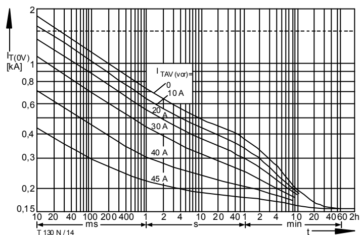
Bild / Fig. 14 Überstrom / Overload on-state current I_{T(OV)} = f(t) Luftselbstkühlung / Natural air-cooling, t_A = 45^\circ\text{C} Kühlkörper / Heatsink: K0.11-M12-A Parameter: Vorlaststrom / Pre-load current I_{TAV(vor)}
