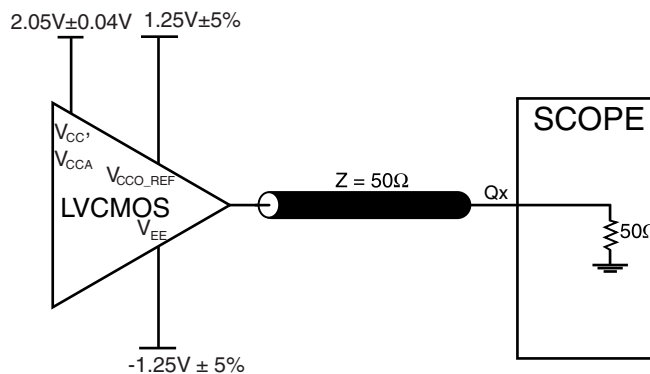
3.3V CORE/2.5V REF_CLK OUTPUT LOAD AC TEST CIRCUIT
