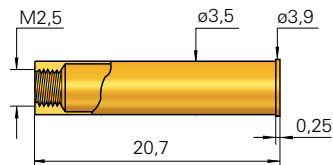
KS-500 M2,5
