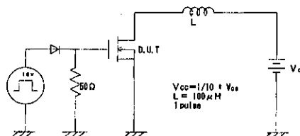
図1 測定回路 Test circuit
