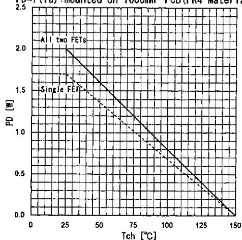
電力損失 Power dissipation
