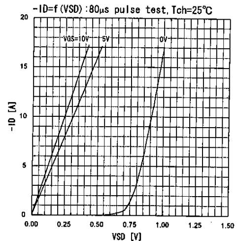
リバースダイオード順特性 Typical forward characteristics of reverse diode
