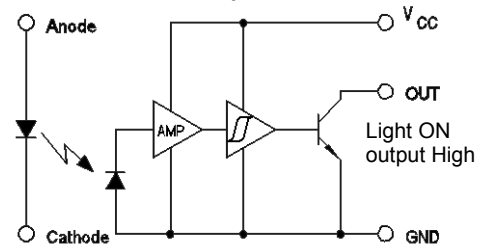
OPB917BOCZ Open-Collector
