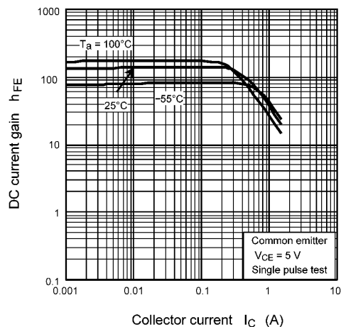
Fig. 7.2 h_{FE} - I_C
