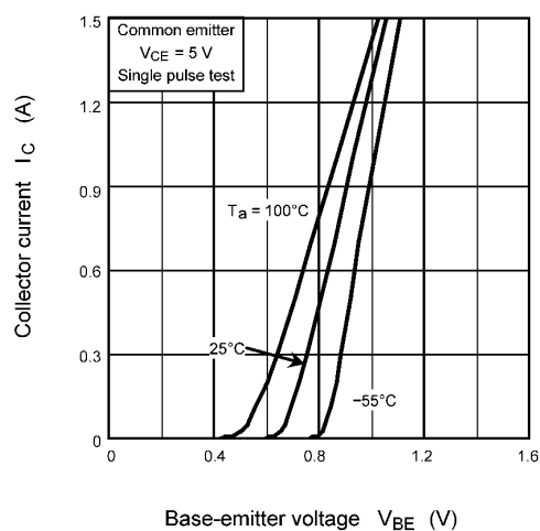
Fig. 7.5 I_C - V_{BE}
