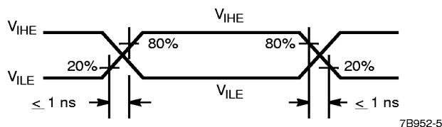
(d) ECL Input Test Waveform
