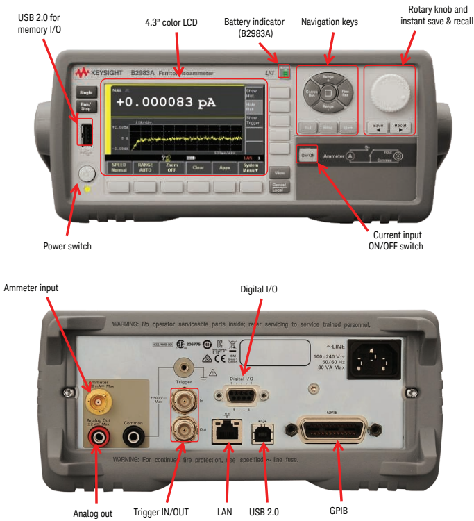
B2981A, B2983A Femto/Picoammeter
