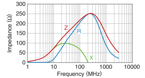
KPZ1608SHR221ATD25
