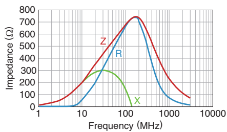
KPZ1608SHR601ATD25
