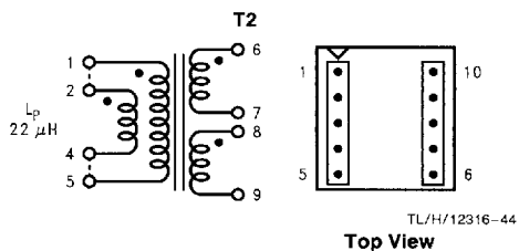
FIGURE 30. Schott 67140860
