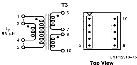
FIGURE 31. Schott 67140920
