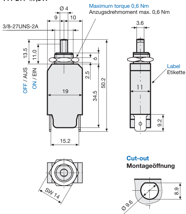
T11-211 ≤7,5 A
