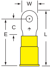
13-4S-NB Stud Size 4 Wire Range 12-10
