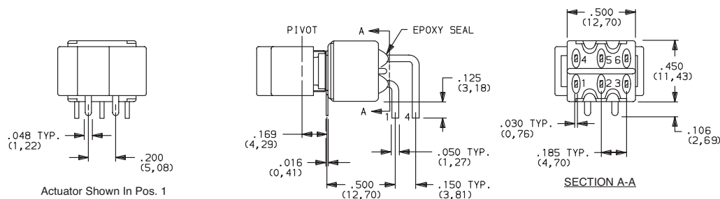
Actuator Shown In Pos. 1
