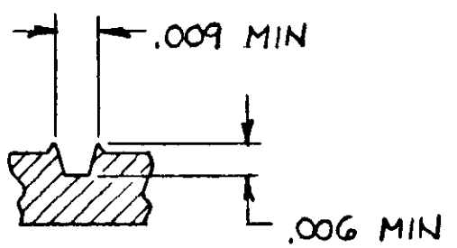
SECTION B-B TYP SERRATION
