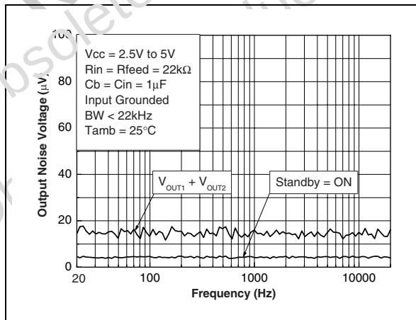
Fig. 25 : Noise Floor
