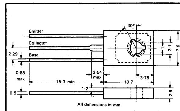
SOT-32
