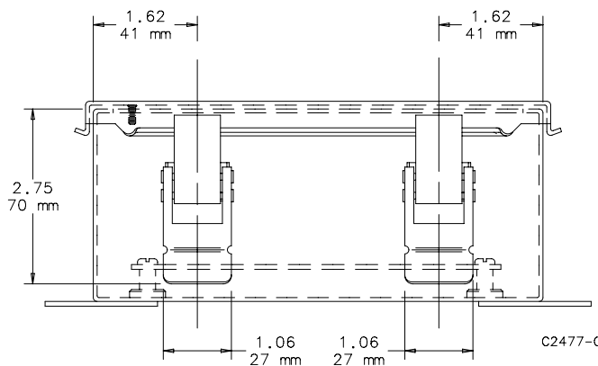
A ≥ 8.00 (203mm)
