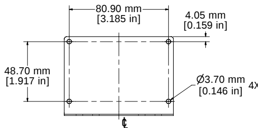
FLANGE
