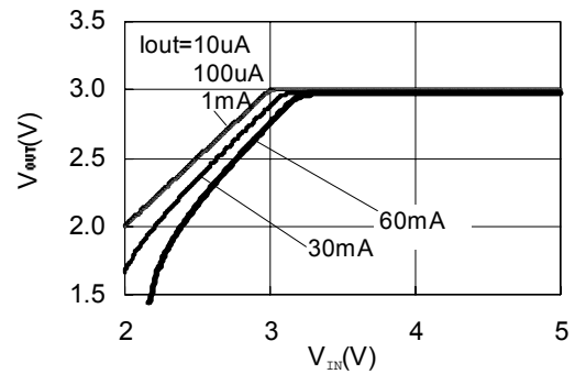
S-814A30A (Ta=25°C)
