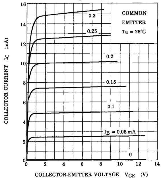
I_C - V_{CE}
