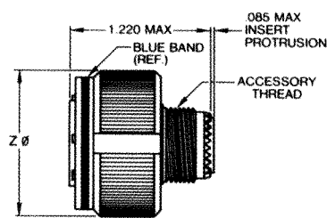
RFI PLUG
